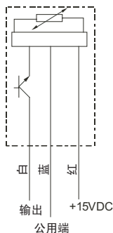
HX-9100-8001 接线图
